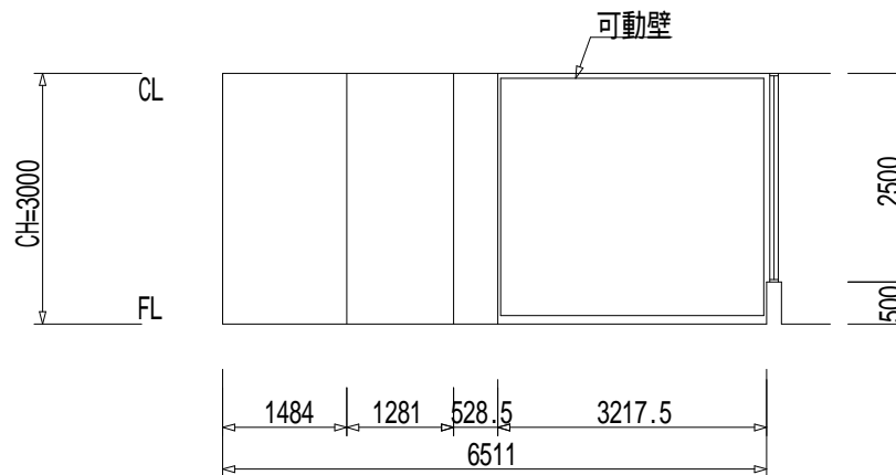
<展开図 D>
